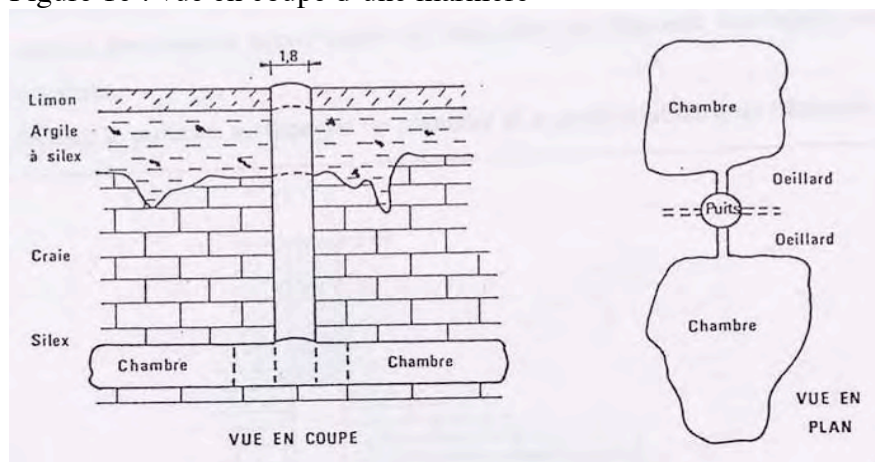
Figure 10 : vue en coupe d'une marnière
