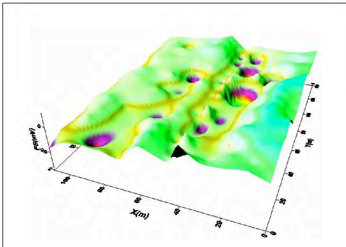
Figure 16 : Profil 3D de polarisation spontanée dans un thalweg du secteur de Bouville
