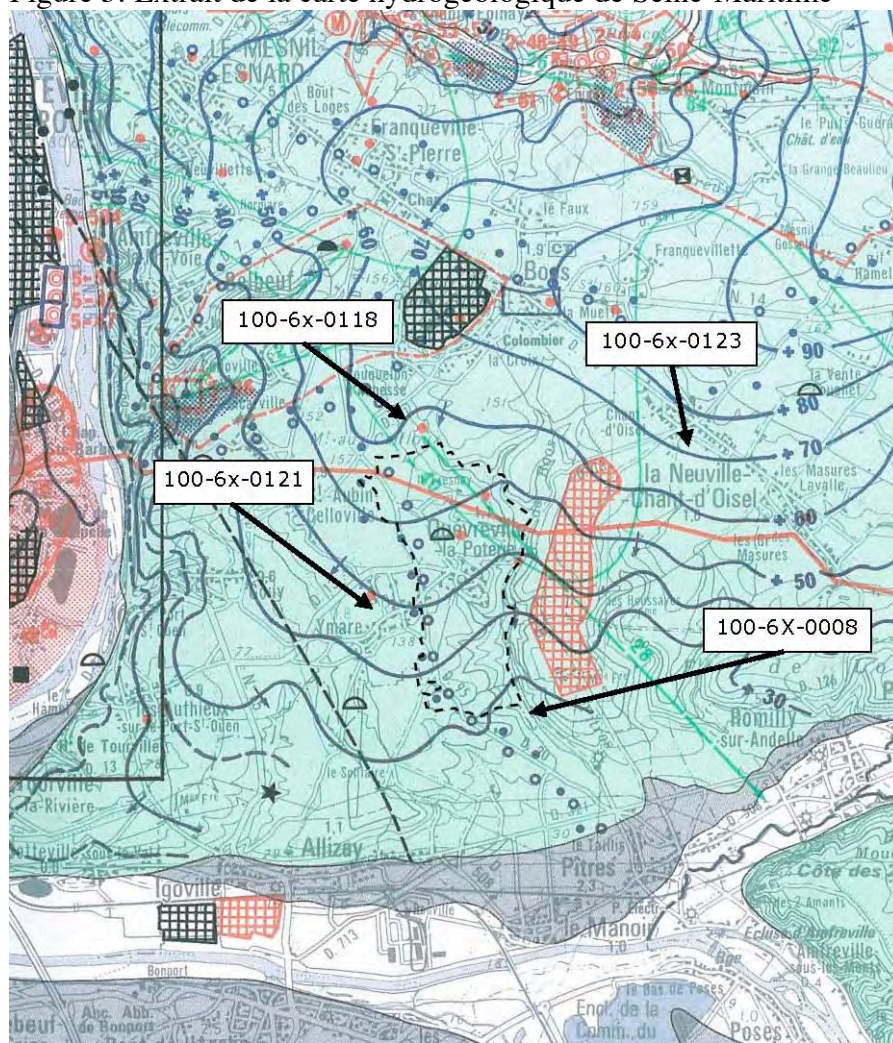
Figure 5: Extrait de la carte hydrogéologique de Seine-Maritime
