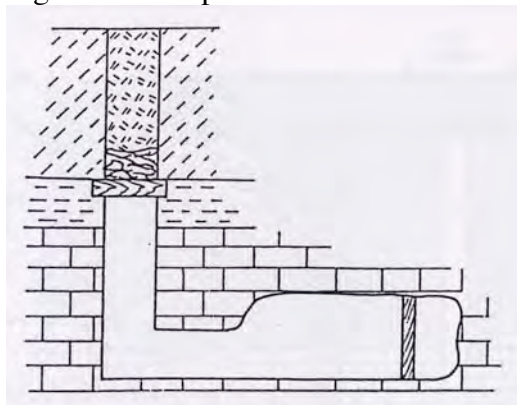
Figure 11 : coupe d'une marnière abandonnée
