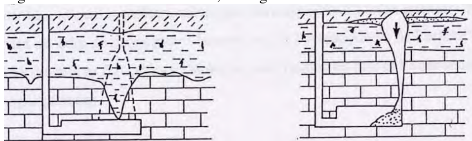
Figure 13 : Formation d'un fontis, vidange d'une racine d'altération
