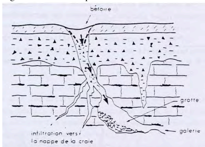
Figure 12 : vue en coupe d'une bétaire
